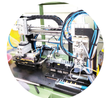
치간칫솔 캡 자동조립
