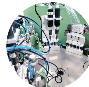
치간칫솔 자동 조립 설비
