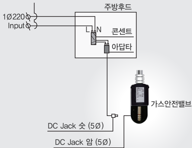
가스안전밸브전원결선회로도
