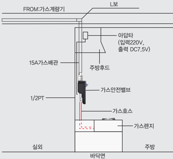
가스안전밸브전원결선회로도
